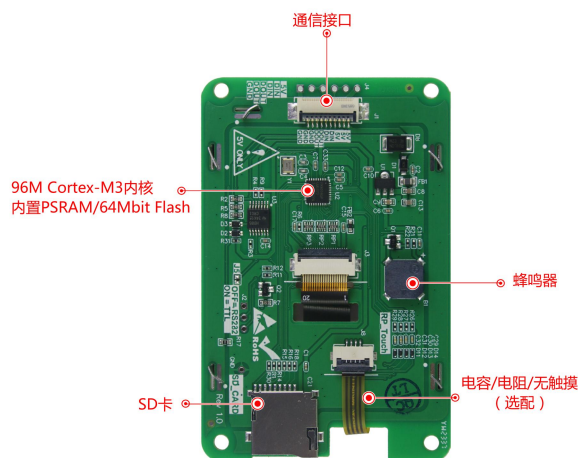
图 1-2 硬件配置图
